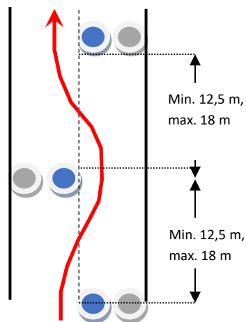
Retardér na dostatočne širokej ceste
