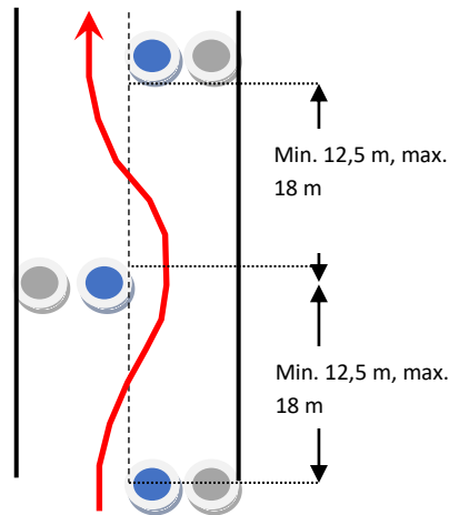
Retardér na dostatočne širokej ceste
